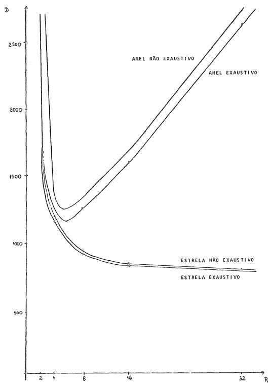
FIGURA 4 - Retardo versus número de Redes Interligadas Disciplinas Exaustiva e Não Exaustiva
