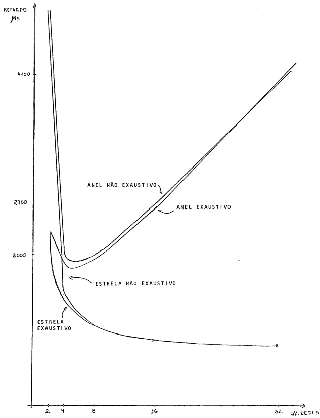
FIGURA 3 - Retardo versus número de Redes Interligadas Disciplinas Exaustiva e Não Exaustiva
