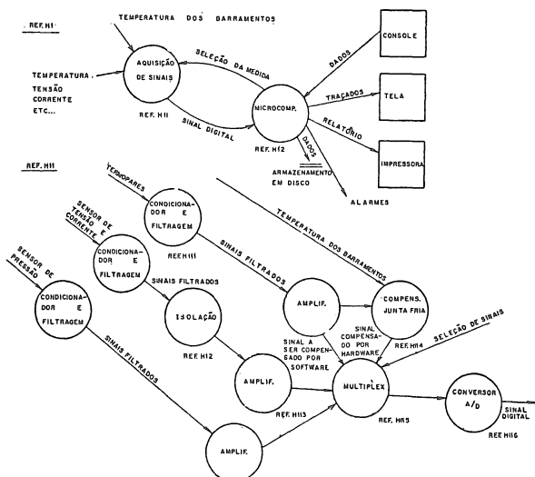
Figura 3: Diagrama de fluxo de informação para parte do hardware do sistema
