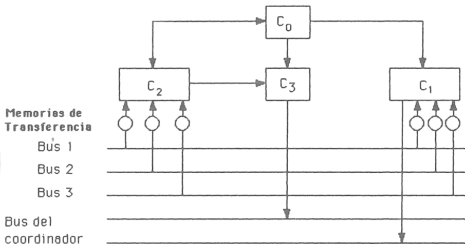
Fig. 5 Subsistema Coordinador.
