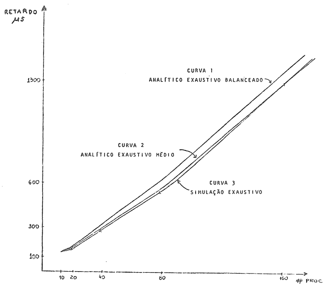
FIGURA 2 - Tempo Médio de espera em uma Rede versus o número de Processadores na rede p/ Disciplina Exaustiva
