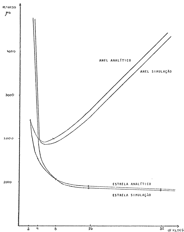
FIGURA 1 = Retardo versus número de Redes Interligadas utilizando a Disciplina não Exaustiva
