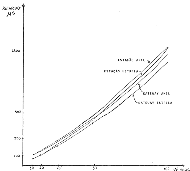
FIGURA 5 - Tempo de Espera nas Estações Usuárias e nos Gateways em função do número de Processadores na Rede
